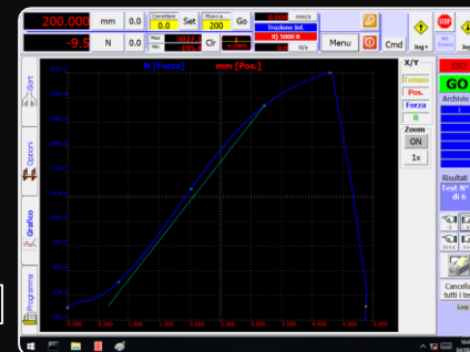
TENSILE (BREAK)
